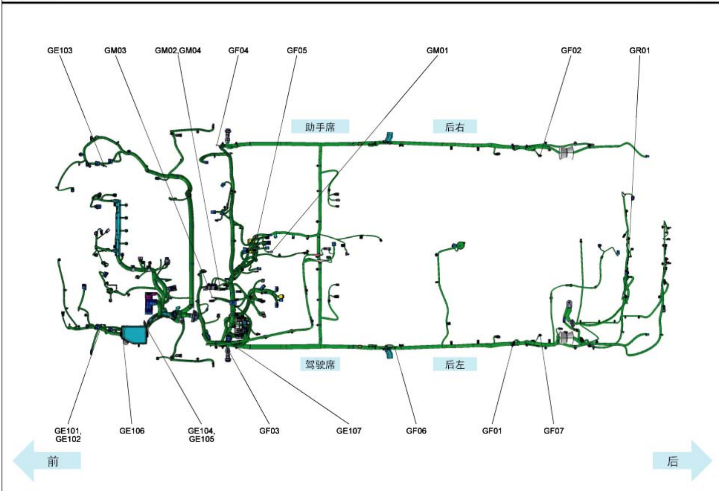
搭铁点(1)
